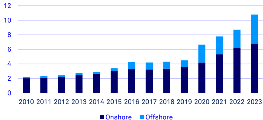
Opgesteld vermogen windenergie Nederland (GW)
