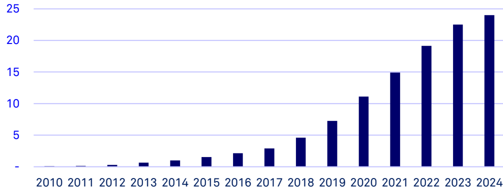
Opgesteld vermogen zonnestroom Nederland (GW)
